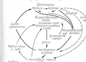
Рис. 6. Круговорот фосфора (по Одуму, 1975)
