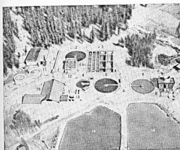
Рис. 1.5.1. Очистное сооружение вблизи г. Южное
