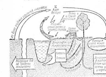
Рис. 5. Схема круговорота азота (по Перельману, 1971)
