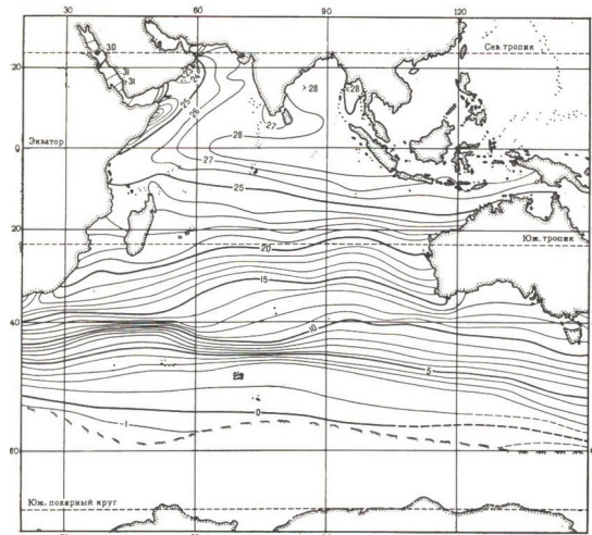
Рис. 6. Температура воды на поверхности океана в августе (в градусах С); прерывистые волнистые линии — кромка дрейфующих льдов
